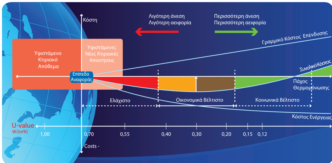
Ανάλυση βέλτιστης τιμής θερμομόνωσης [9]
