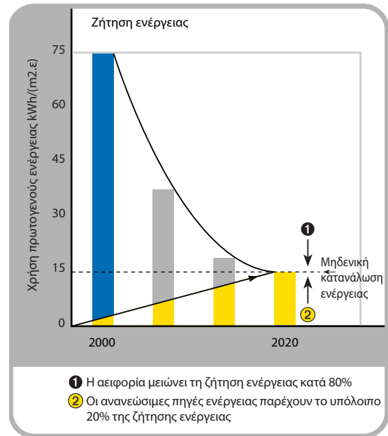
Προσέγγιση για τον Σχεδιασμό Κτιρίων με Μηδενική Κατανάλωση Ενέργειας
