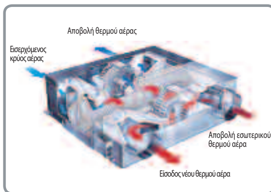
Εικ. Αρχή της λειτουργίας ανάκτησης θερμότητας σε ένα σύστημα εξαερισμού [9]
